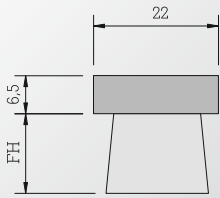
FBL 1310
