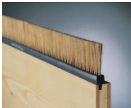
Zum Einstecken in Nuten Inserted into a groove Pour insérer dans des rainures
