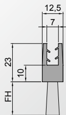
FBL 1341
