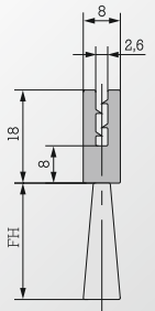
FBL 1310
