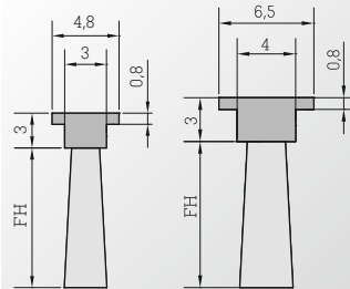
FBL 1248 / 1265
