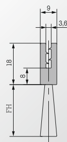
FBL 1320
