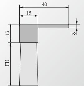
FBL 4005
